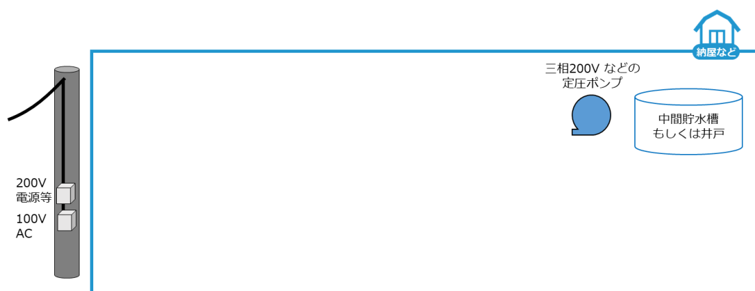
図 2-1 原水・ポンプと電源の施工概要図
